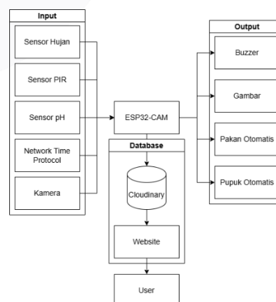
Gambar 1 Diagram Blok Sistem
