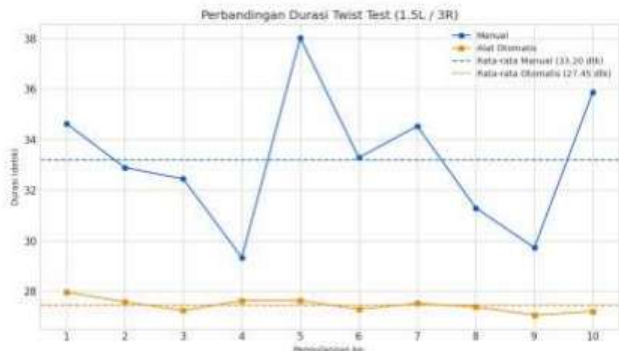
Gambar 12 Perbandingan Durasi Twist 1.5 – 3 Putaran.
