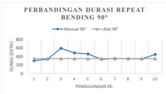
Gambar 9 Grafik Perbandingan Durasi Pengujian Repeated Bending .
