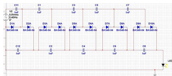
GAMBAR 5 (Skematik rangkaian rectifier)
