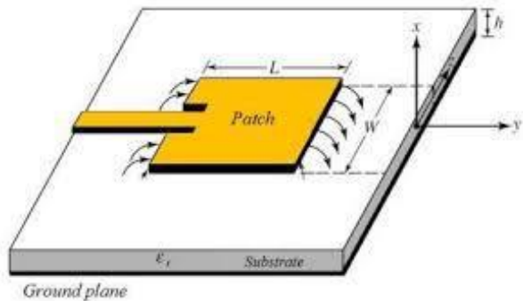
GAMBAR 1 (Antena Mikrostrip)
