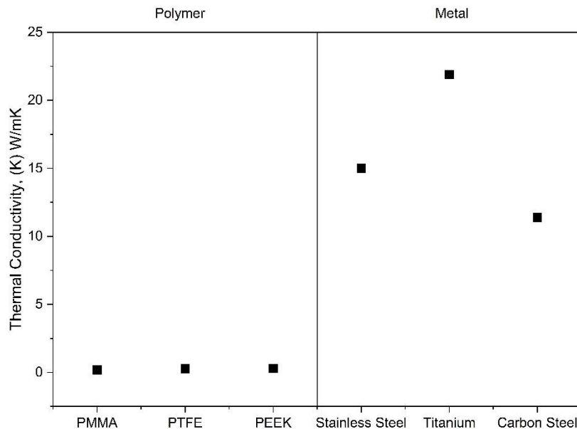
Gambar I-1. Perbandingan konduktivitas termal polimer dengan logam. Polimer menunjukkan konduktivitas termal yang jauh lebih rendah dibandingkan logam.
