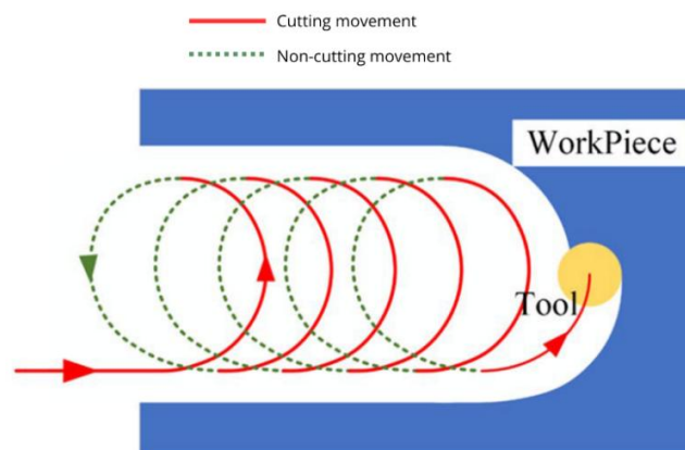
Gambar I-2. Jalur mata pahat dengan bentuk kurva trochoid pada proses pembuatan slot (dimodifikasi, dari Zhang et al., 2024 © Author)
