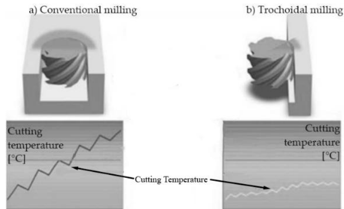
Gambar I-3. Perbandingan suhu pemotongan pada proses permesinan. a) Milling Konvensional b) Trochoidal Milling (Dimodifikasi, dari Waszczuk, 2024 © Author)
