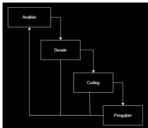
Gambar 1-1 Tahap Metode Waterfall
