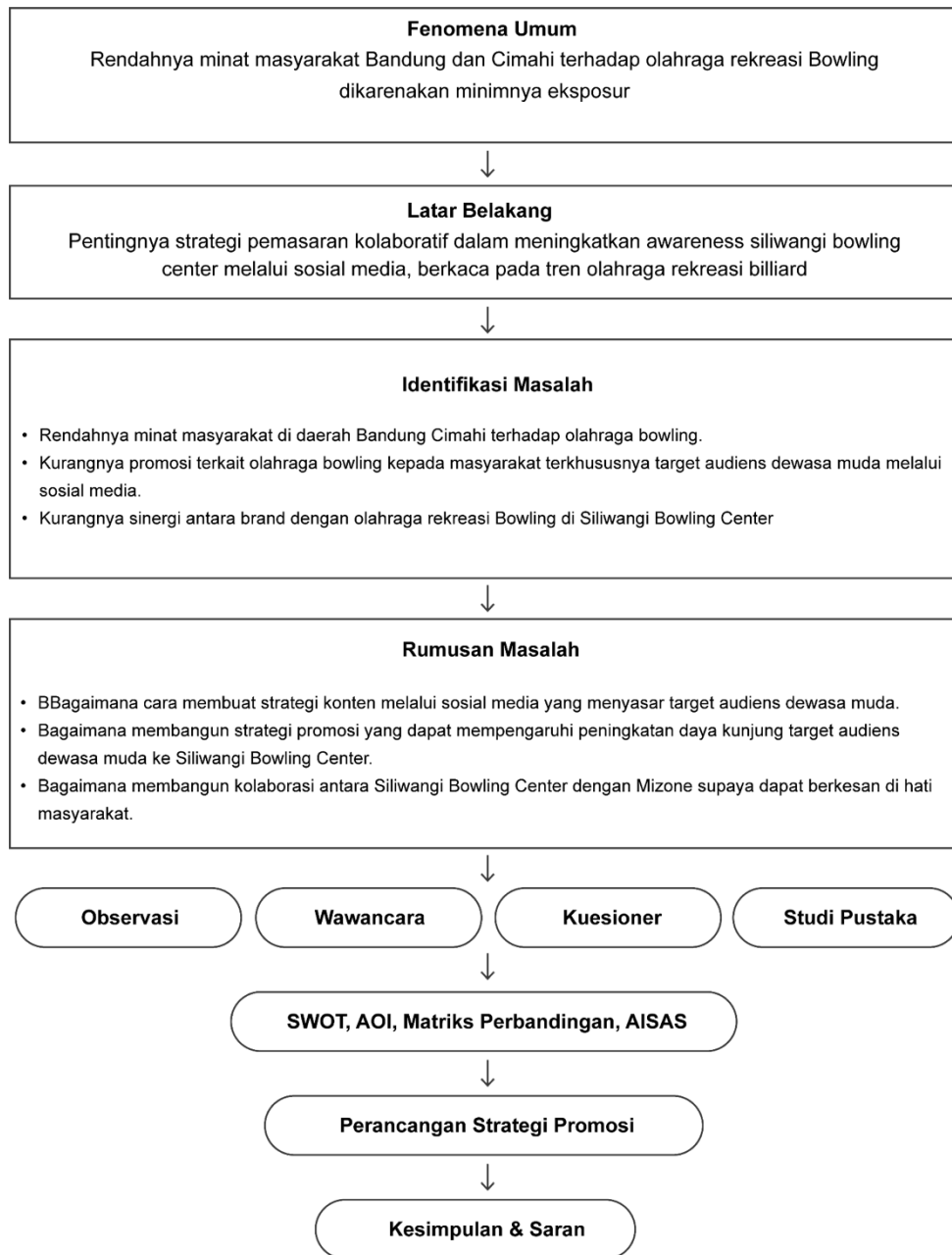
Gambar 1.1 Kerangka Perancangan
