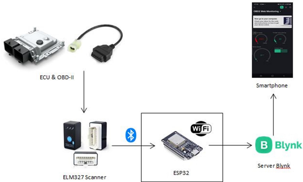
Gambar 3. 1 Perancangan Sistem
