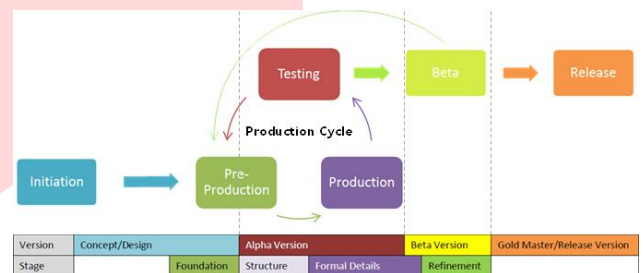
GAMBAR 1. Tahap GDLC [10]
