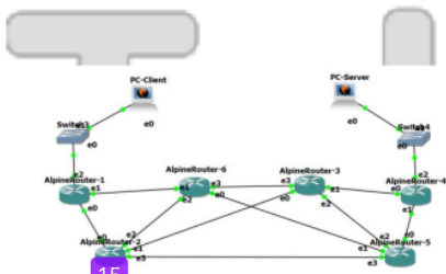
Gambar 3. 2 Topologi Jaringan
