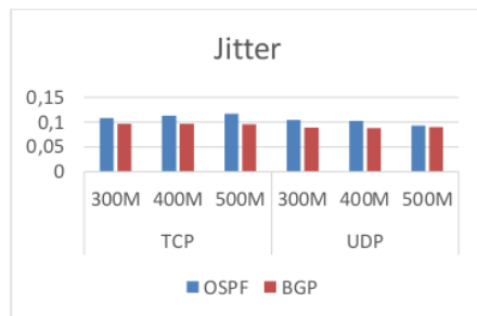
Gambar 4. 6 grafik jitter
