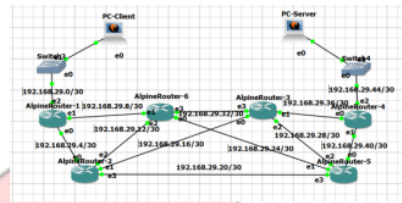
Gambar 3. 3 Topologi dan alamat Ip
