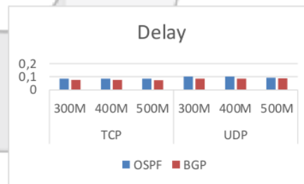
Gambar 4. 5 grafik delay
