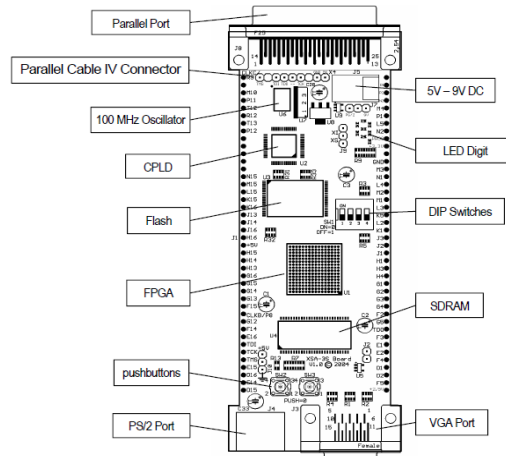
Gambar 3.2 Pengaturan komponen pada Board XSA-3S1000.
